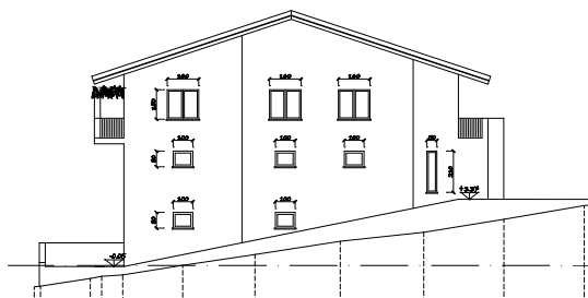
Nuovo Edificio prospetto EAST
